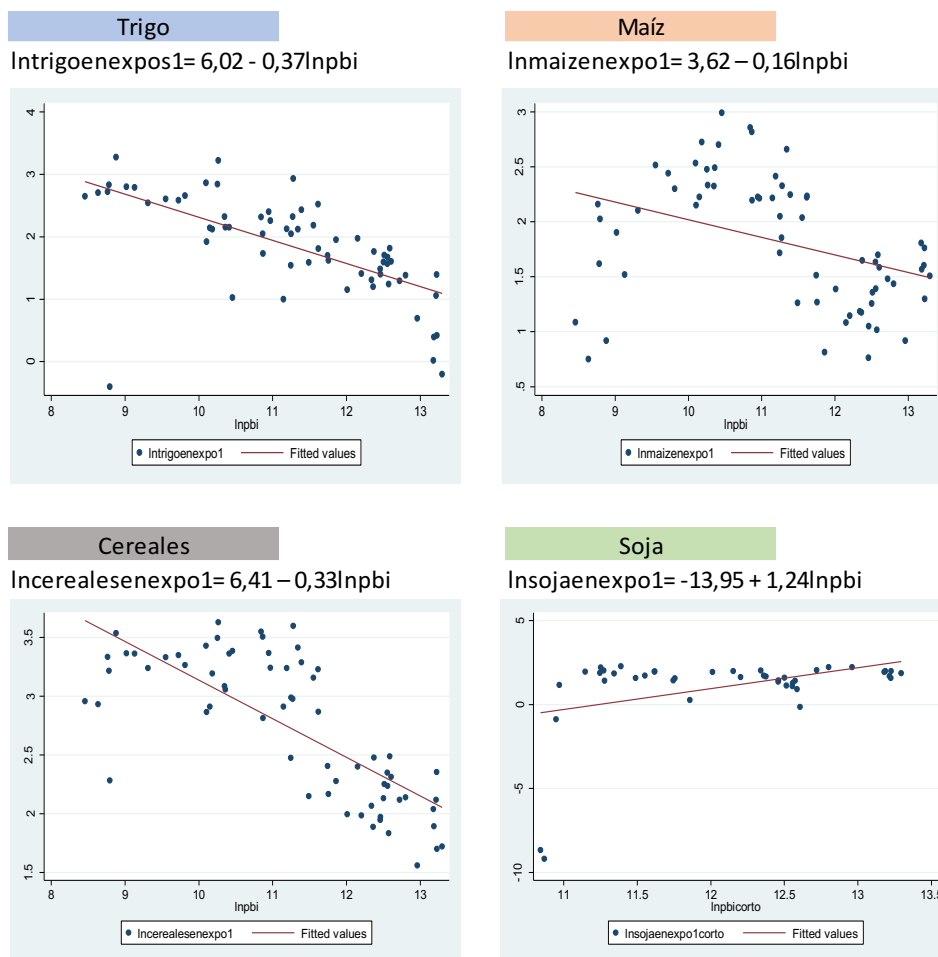
Gráfico 5. Regresión lineal por Mínimos Cuadrados Simples Graphic 5. Linear regression by Minimum Simple Squares
